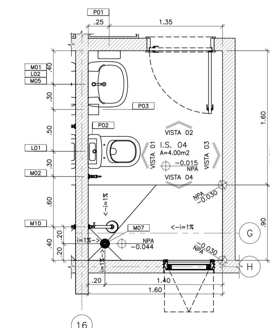
UNIDADE DE PRONTO ATENDIMENTO – PORTE 2 I.S. 04 ESCALA: 1:25
