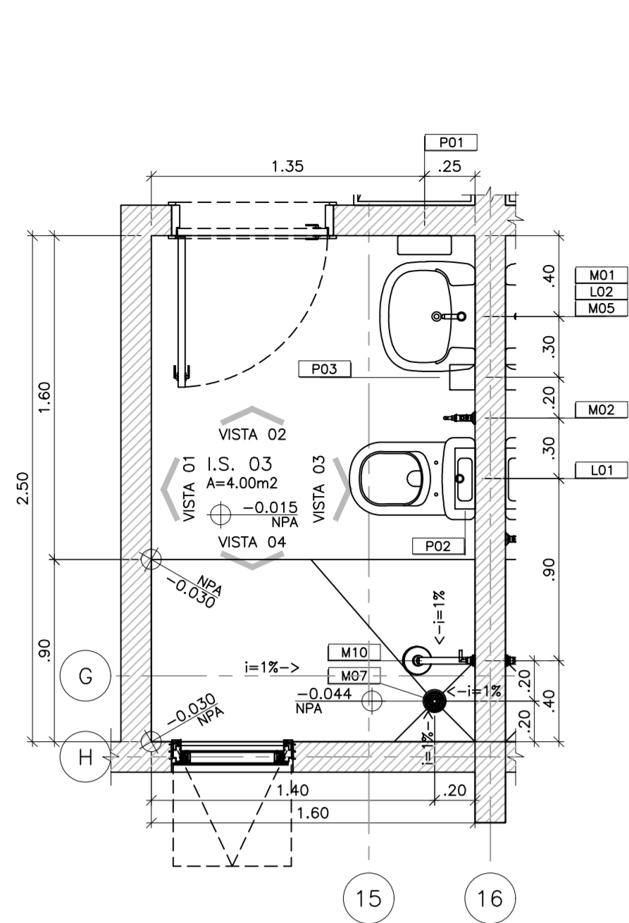
UNIDADE DE PRONTO ATENDIMENTO – PORTE 2 I.S. 03 ESCALA: 1:25
