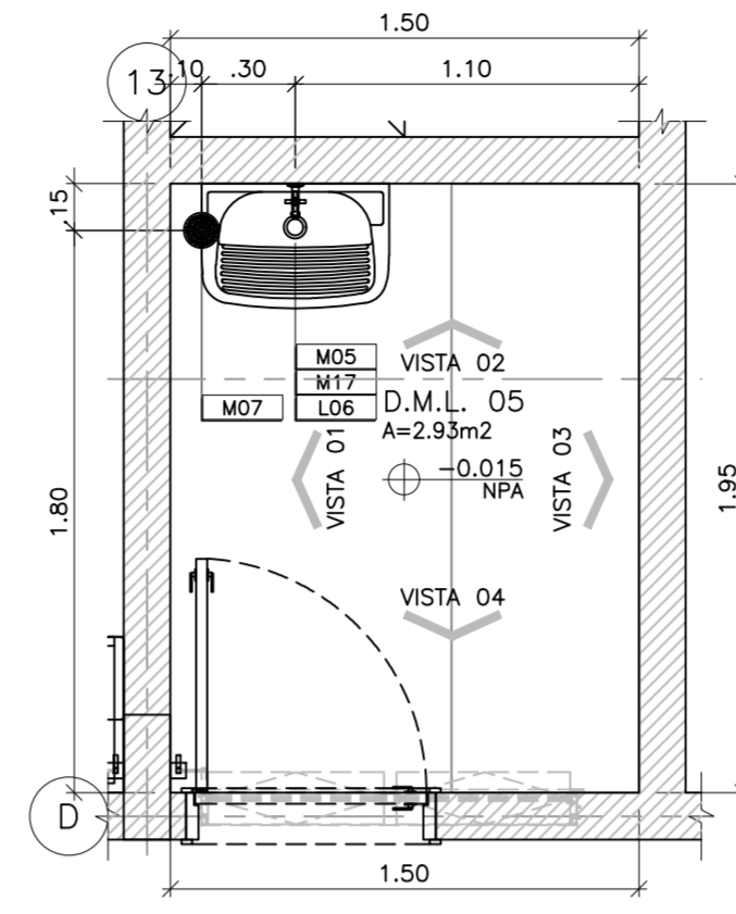
UNIDADE DE PRONTO ATENDIMENTO – PORTE 2 D.M.L. 05 ESCALA: 1:25
