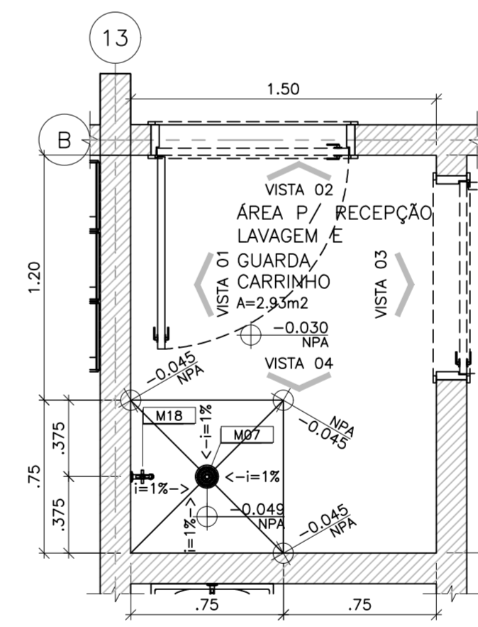
UNIDADE DE PRONTO ATENDIMENTO – PORTE 2 ÁREA P/ RECEPTÃO, LAVAGEM E GUARDA CARRINHO ESCALA: 1:25
